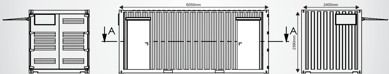
MODULO HABITABLE SANITARIO 20 pies
