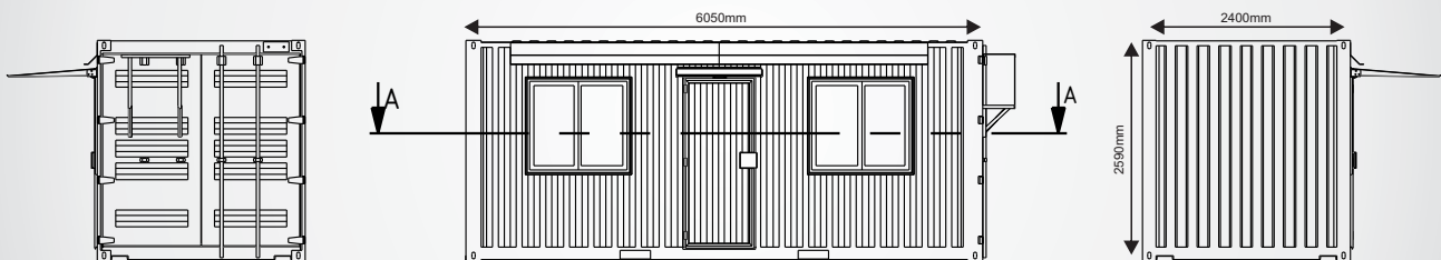
MODULO HABITABLE ESTANDAR 20 pies
