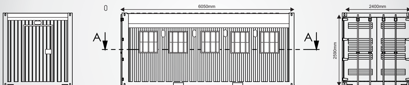
MODULO BOLETERIA ESTANDAR 20 pies
